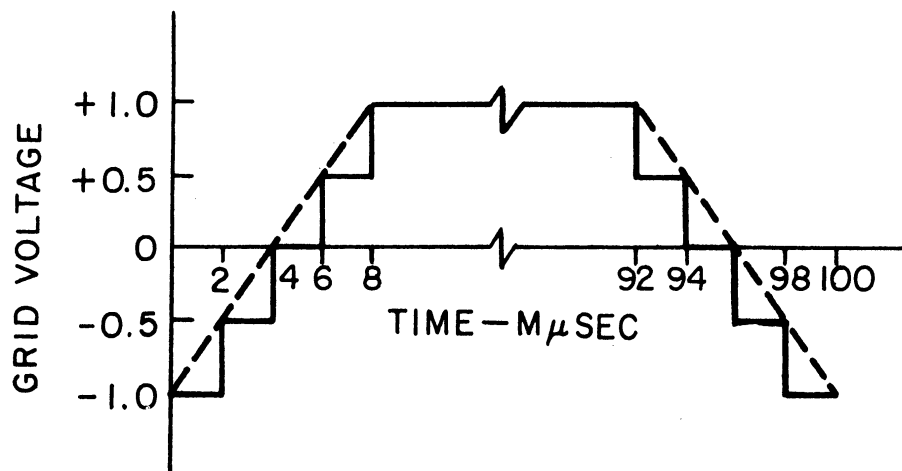
Fig. 1.16. Input signal.
