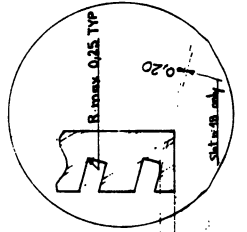
Fig. C-7. LEU CERCA Side Plate
