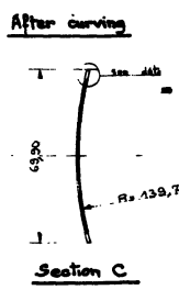
Fig. C-6. LEU CERCA Fuel Plates
