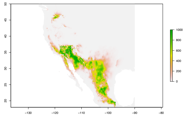
Lampropeltis getula
