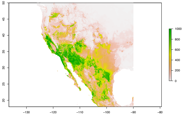
Masticophis flagellum
