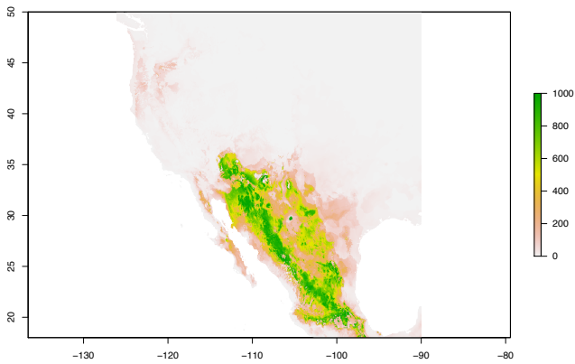
Hypsiglena torquata
