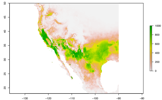
Pituophis catenifer
