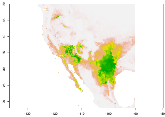
Sonora semiannulata
