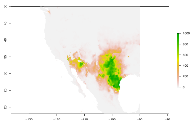
Thamnophis marcianus
