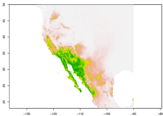
Trimorphodon biscutatus
