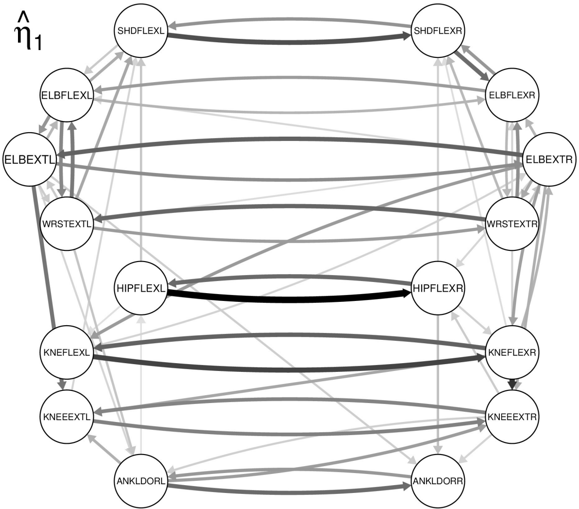
sim_8956_eta1_jan.eps
