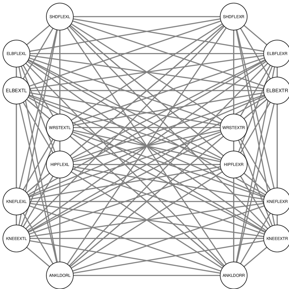
sim_8956_nex1.eps
