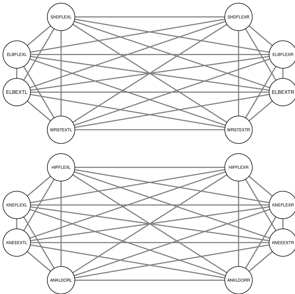
sim_8956_nex2.eps
