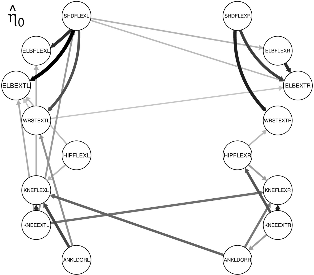
sim_8956_eta0_jan.eps
