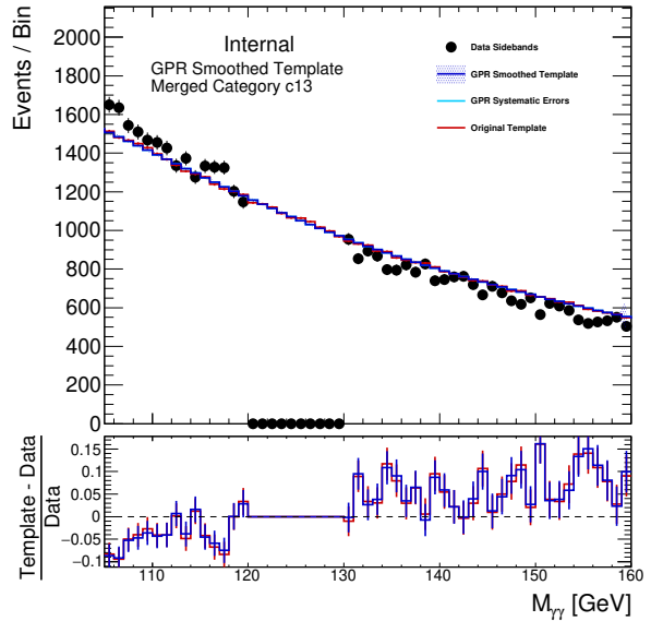
(d) GG2H_GE2J_MJJ_0_350_PTH_60_120_2
