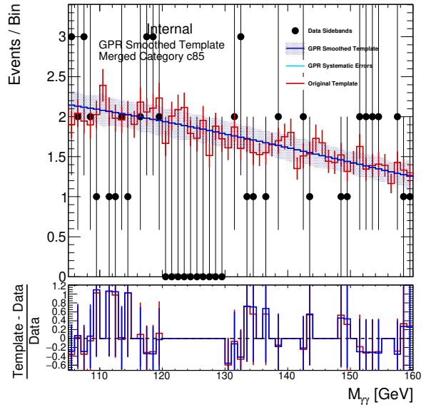
(d) TTH_PTH_120_200_1
