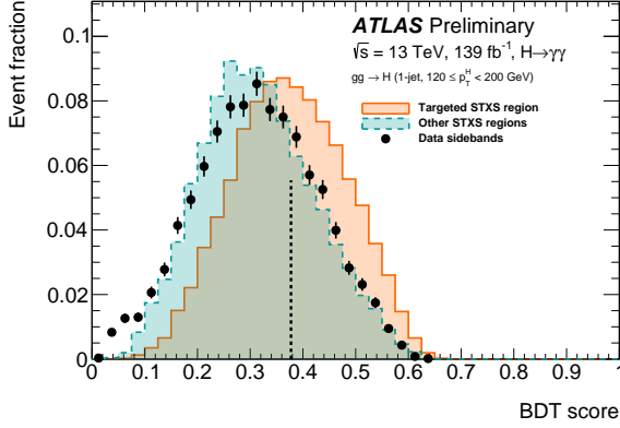
(a) gg \rightarrow H (1-jet, 120 \leq p_T^H < 200 \text{ GeV} )
