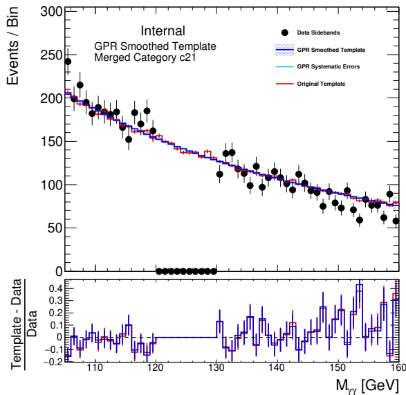
(d) GG2H_GE2J_MJJ_350_700_PTH_0_200_PTHJJ_GT25...2
