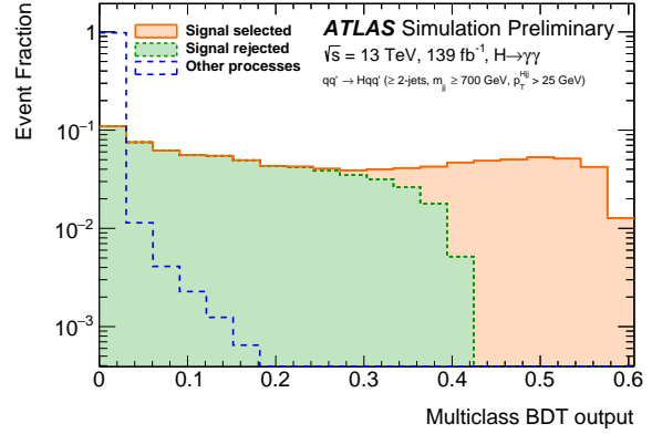
(b) qq \rightarrow Hqq ( \geq 2 -jets, m_{jj} > 700 GeV, p_T^{Hjj} > 25 GeV)
