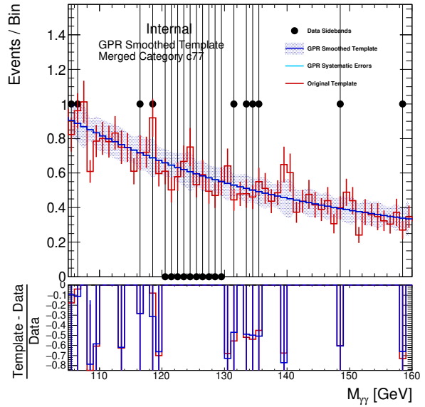
(d) HLL_PTV_150_250_GE1J_0
