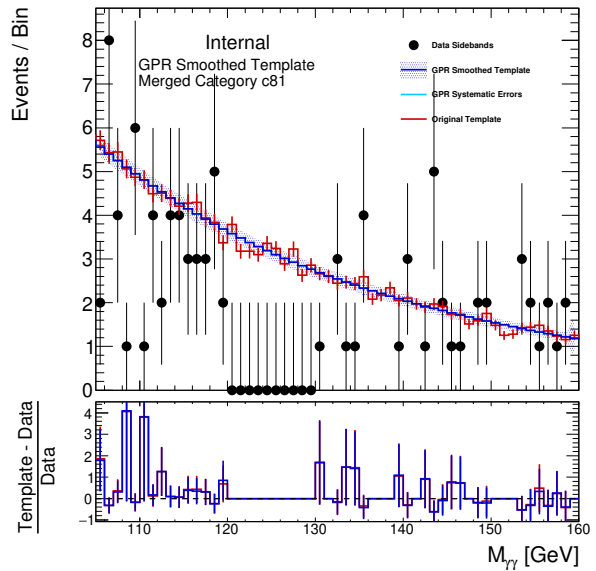
(d) TTH_PTH_0_60_1
