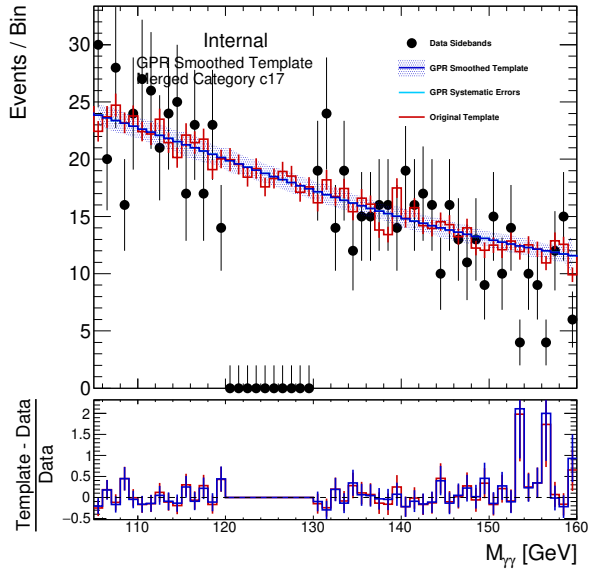
(d) GG2H_GE2J_MJJ_350_700_PTH_0_200_PTHJJ_0_25_1
