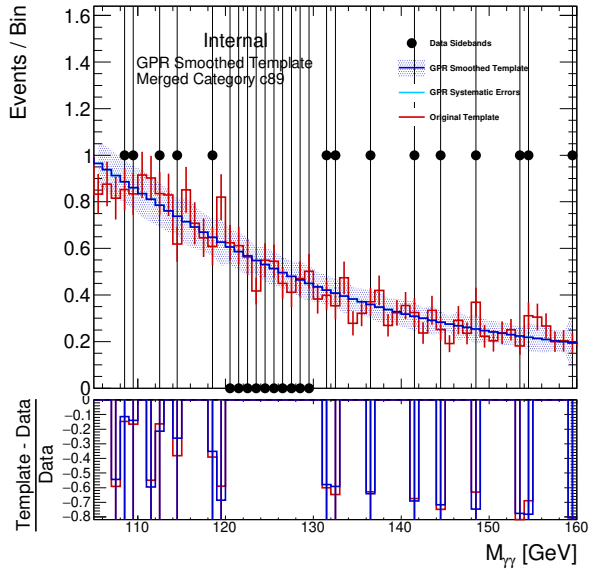
(d) TWH_0
