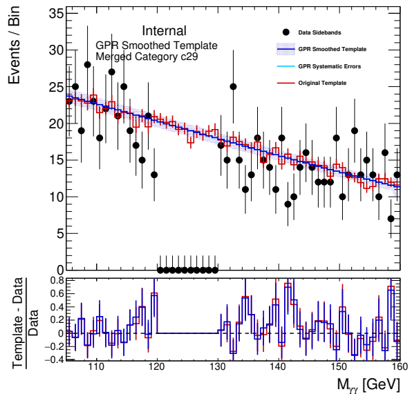
(d) GG2H_PTH_200_300_1
