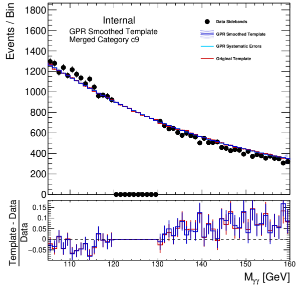
(d) GG2H_GE2J_MJJ_0_350_PTH_0_60_1
