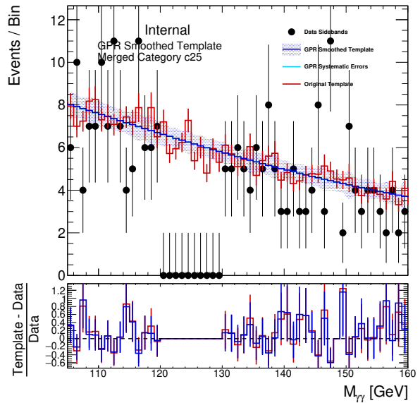
(d) GG2H_GE2J_MJJ_GT700_PTH_0_200_PTHJJ_GT25_0
