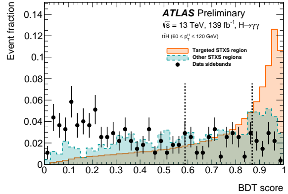
(d) t\bar{t}H ( 60 \leq p_T^H < 120 \text{ GeV} )
