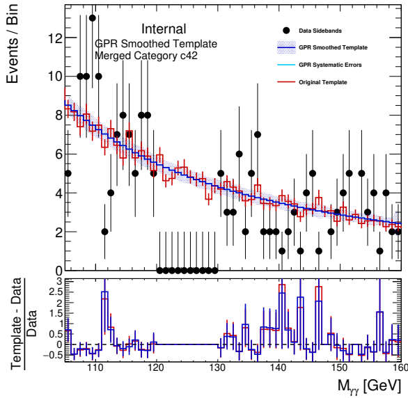
(a) QQ2HQQ_1J_2
