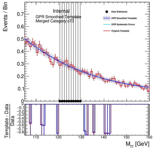
(d) HLL_PTV_0.75_0
