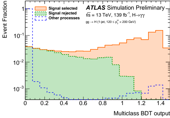
(a) gg \rightarrow H (1-jet, 120 \leq p_T^H \leq 200 GeV)
