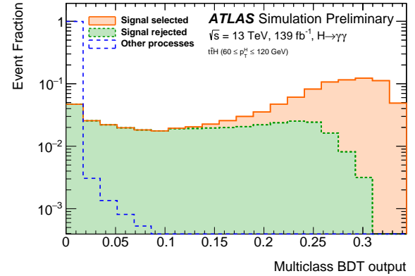
(d) t\bar{t}H ( 60 \leq p_T^H < 120 GeV)
