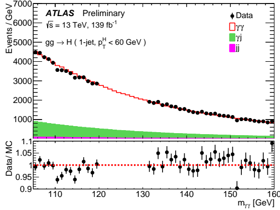
(a) gg \rightarrow H (1-jet, p_T^H < 60 GeV)
