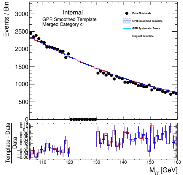
(d) GG2H_1J_PTH_60_120
