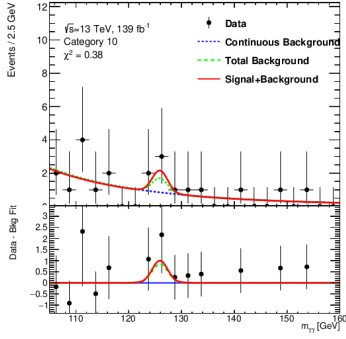
(d) Category 10: m_{\gamma\gamma} (GeV)
