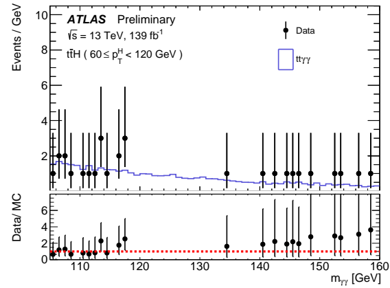
(d) t\bar{t}H ( 60 \leq p_T^H < 120 GeV)
