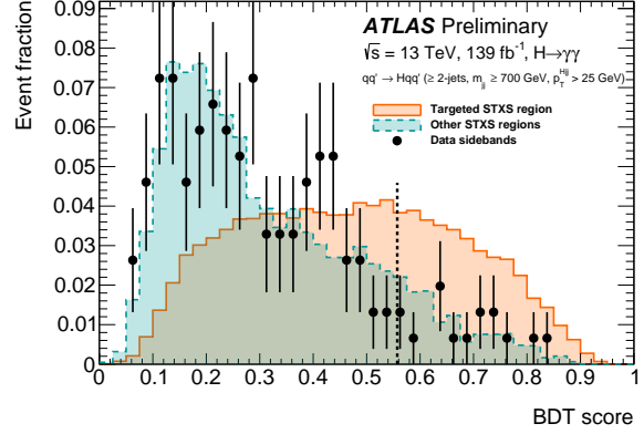
(b) qq \rightarrow Hqq ( \geq 2 -jets, m_{jj} > 700 \text{ GeV}, p_T^{Hjj} > 25 \text{ GeV} )
