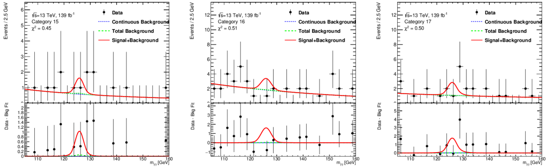
(c) Category 15: m_{\gamma\gamma} (GeV) (d) Category 16: m_{\gamma\gamma} (GeV) (e) Category 17: m_{\gamma\gamma} (GeV)
