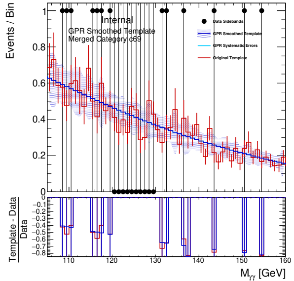
(d) QQ2HLNU_PTV_150_250_0J_0
