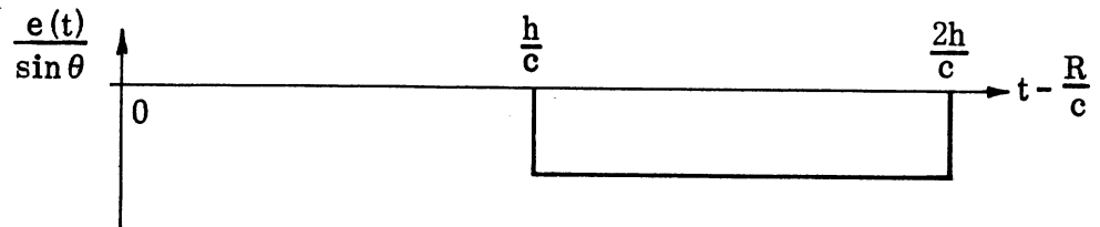
(D) Radiation from Current Step Traveling Inward on -z.
