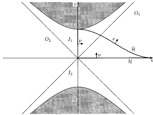
FIG. 1. Kruskal coordinates.
