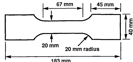
Fig. 1 Tensile specimen.
