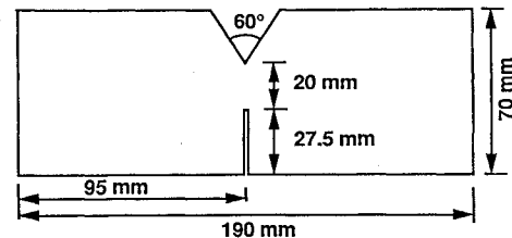
Fig. 2 Fracture-toughness specimen.
