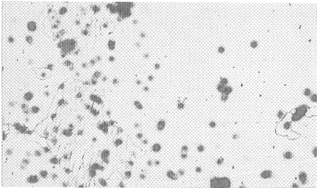
(d) Focus on metal surface. 1,000X. L-84844
